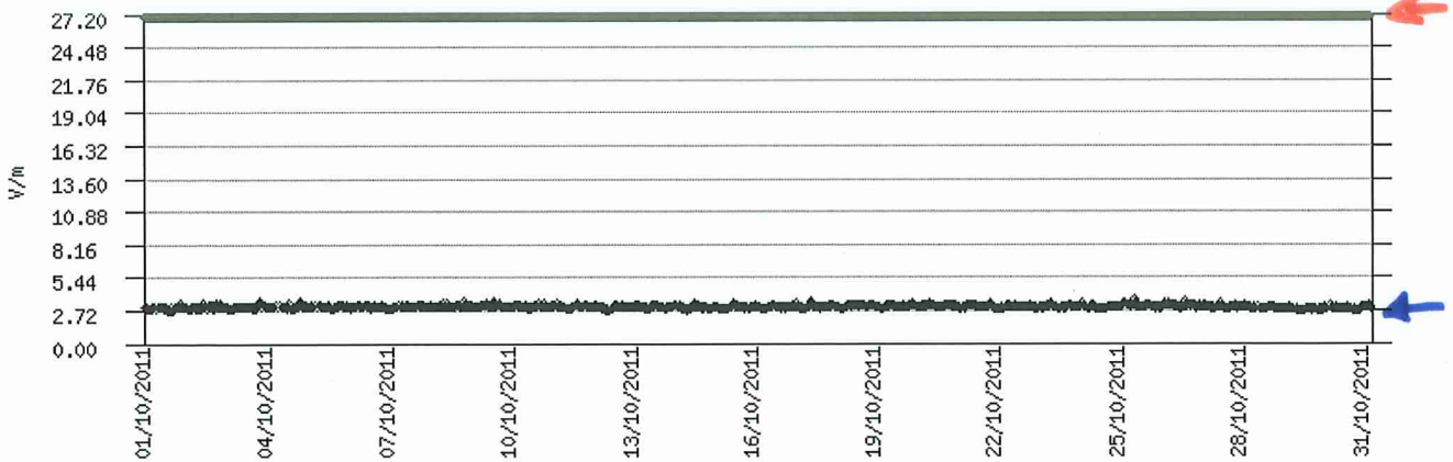
Gràfic comparatiu entre els valors del període (traç blau) i el límit més restrictiu de la normativa (traç vermell).
