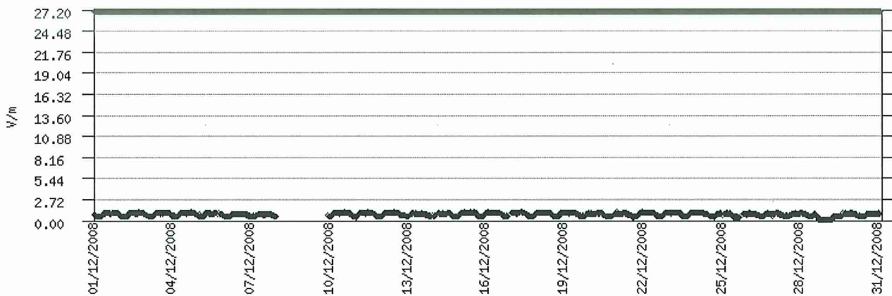
Gràfic comparatiu entre els valors del període (traça blava) i el límit més restrictiu de la normativa (traça vermella). Nota: Els espais en blanc de la gràfica es corresponen amb la manca d'alimentació elèctrica a l'equip SMRF
